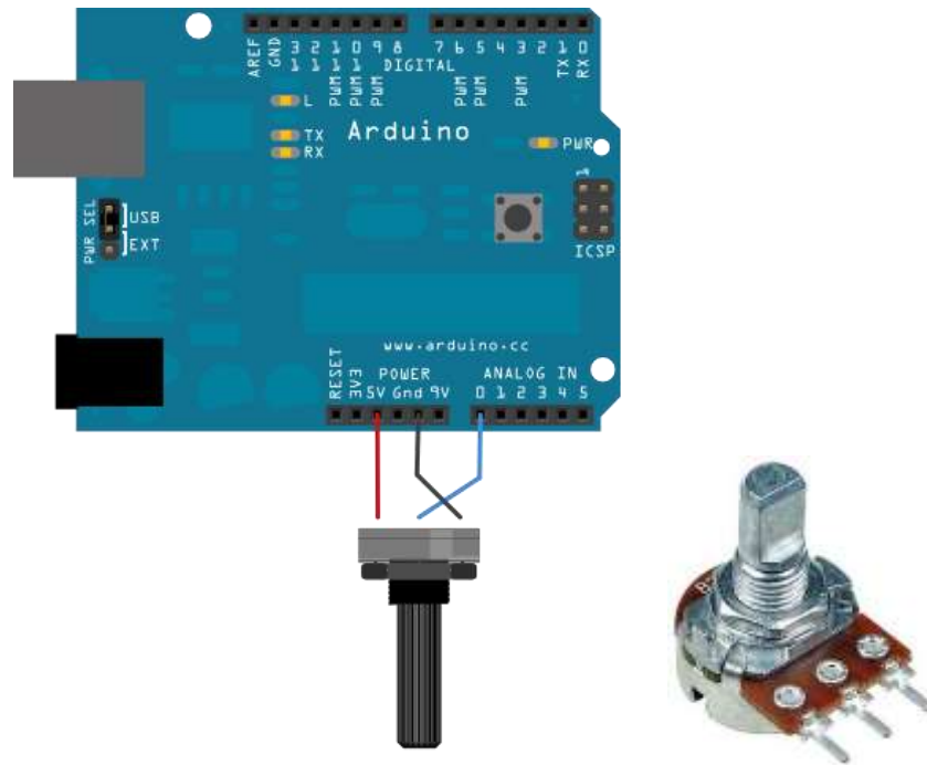
Spajanje potencijometra na analogne ulazne pinove
