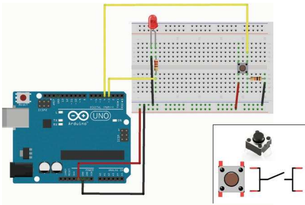
Kontrola LED diode pomoću 4-pinskog prekidača (digitalni ulazni pinovi) (otpornik uz diodu \leq 300\Omega a otpornik uz prekidač 10k\Omega )
