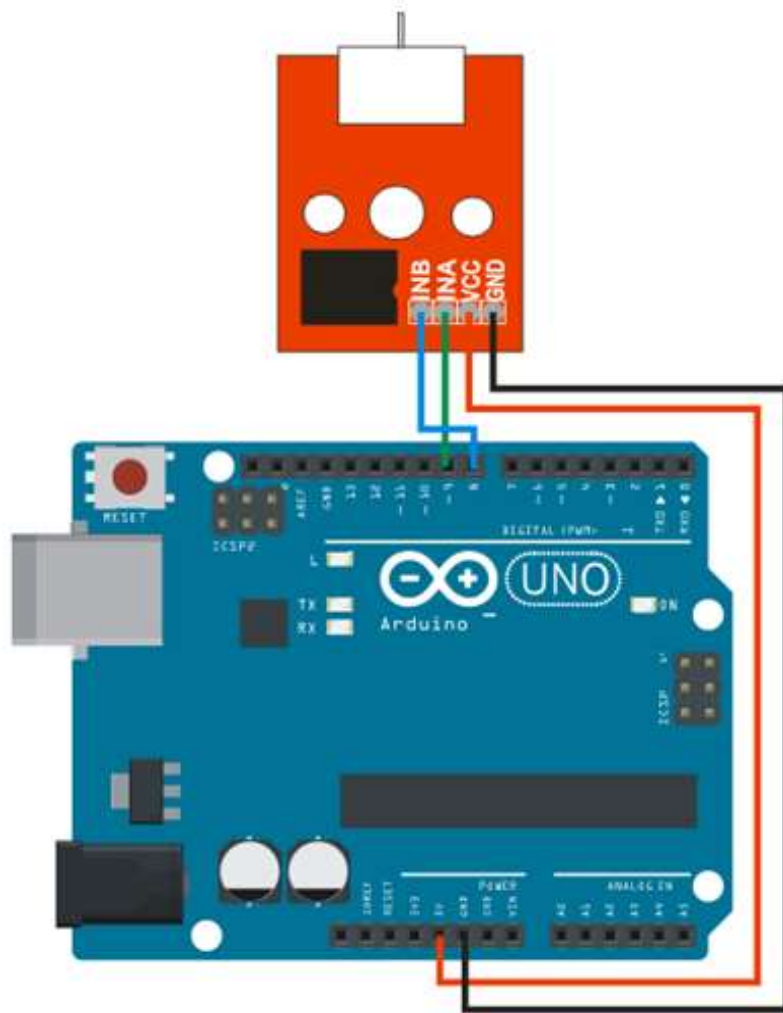
Šema spajanja motora (propelera)
