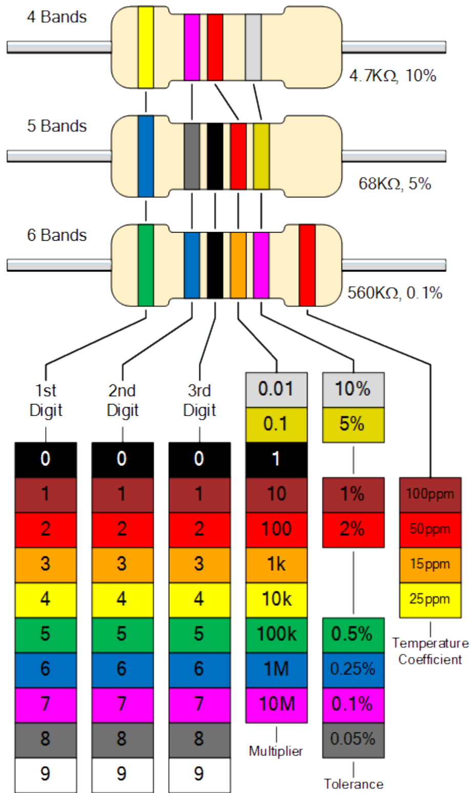
Određivanje vrijednosti otpornika na osnovu boja
