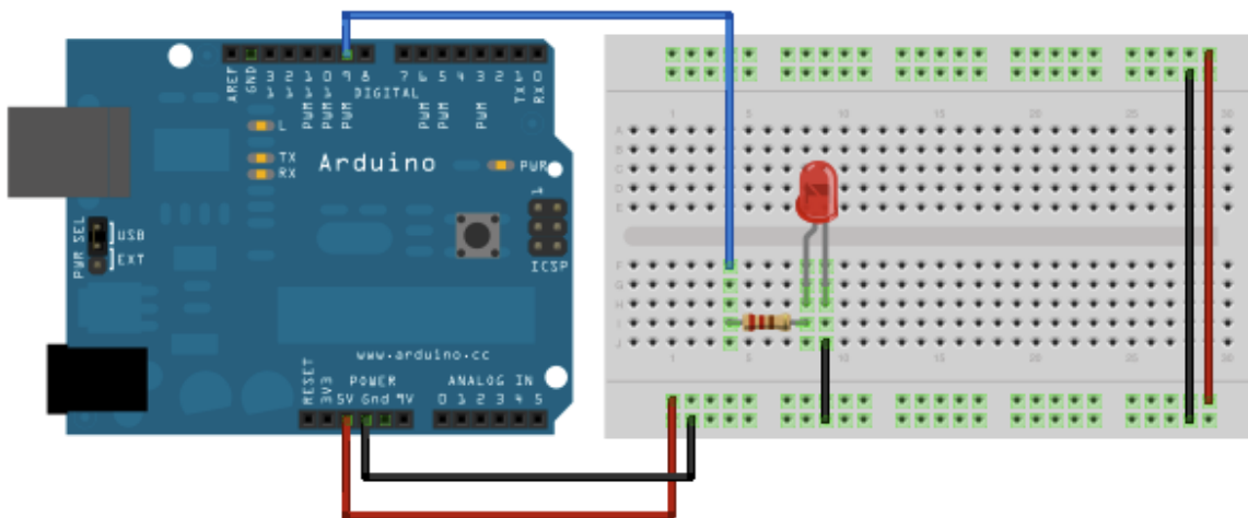
LED svjetleća dioda (otpornik \leq 300\Omega )
